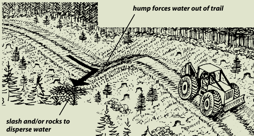
Skid hump.
